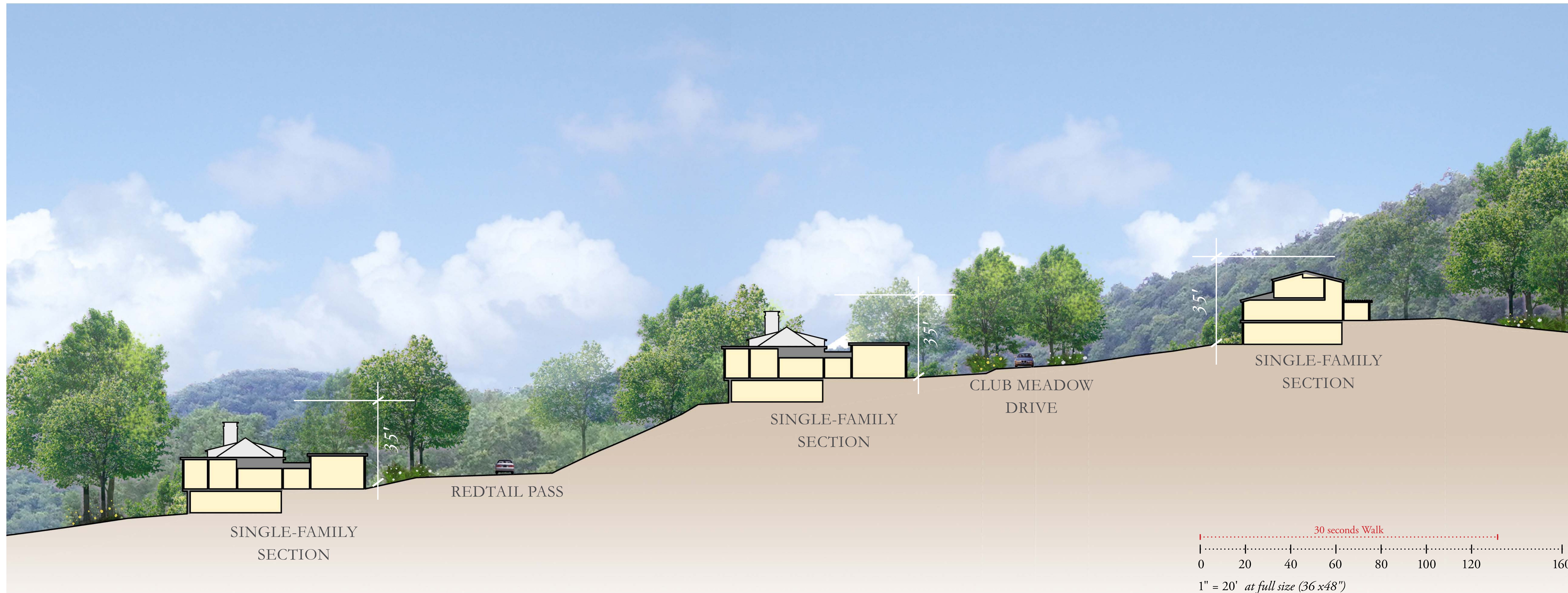
SITE SECTION HH - GOLF VILLAS
