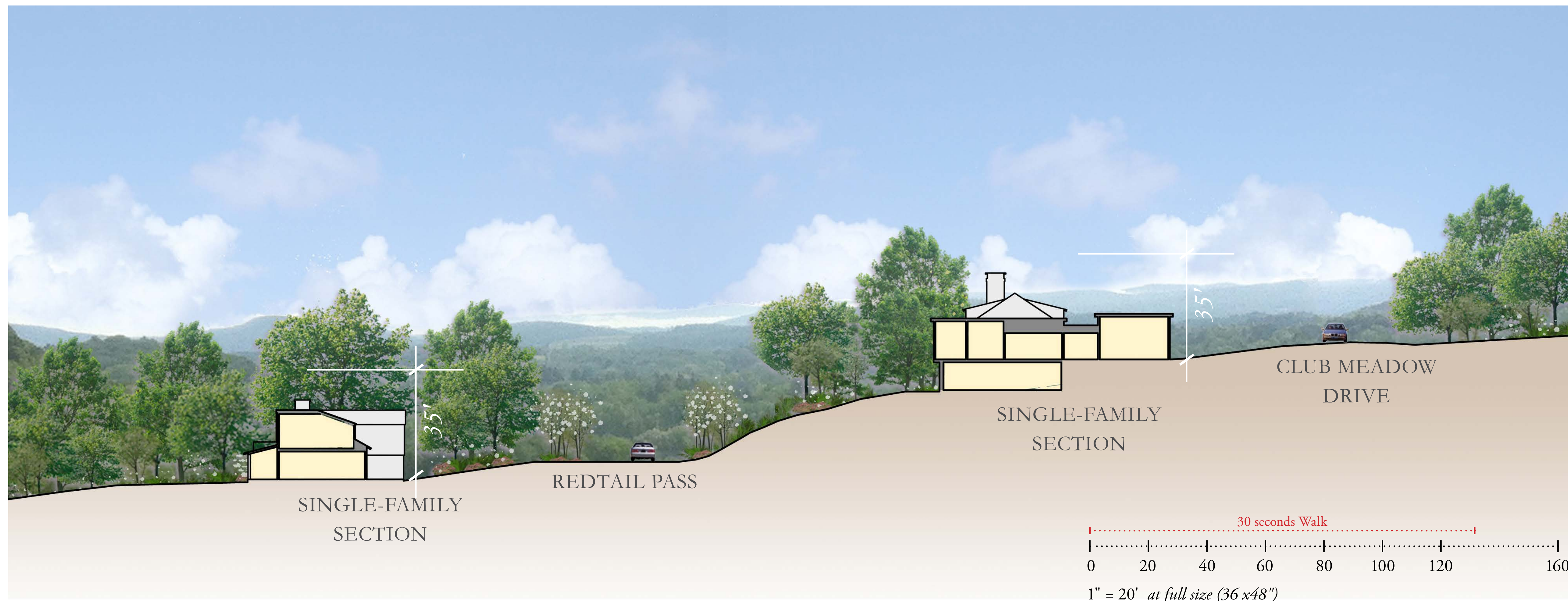
SITE SECTION GG - GOLF VILLAS
